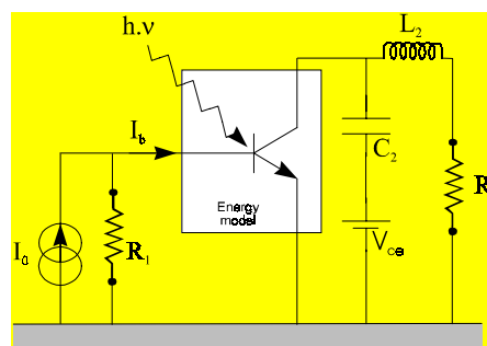
Figure I-2.3b : schéma du modèle électrique complet pour un phototransistor avec une base commandée en courant.
