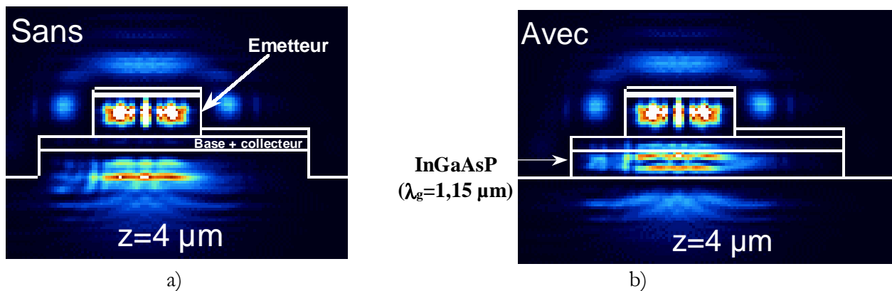
Figure II-4.2 : influence d'une couche de confinement en quaternaire (0,7 \mu\text{m} d'épaisseur) sur la propagation de la lumière (BPM-3D). Puissance optique à une profondeur de 4 \mu\text{m} dans le guide d'onde.
